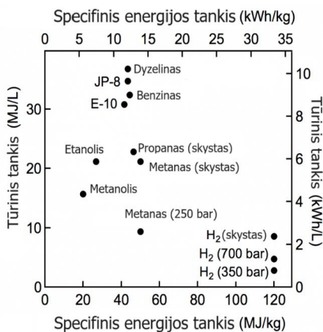
8 pav. Kuro energijos tankių lentelė Šaltinis: sudaryta autoriaus
