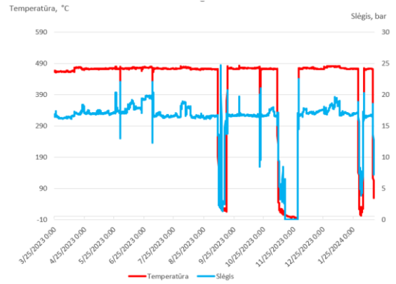
7 pav. Vamzdyno metų trukmės apkrova Šaltinis: sudaryta autorių
