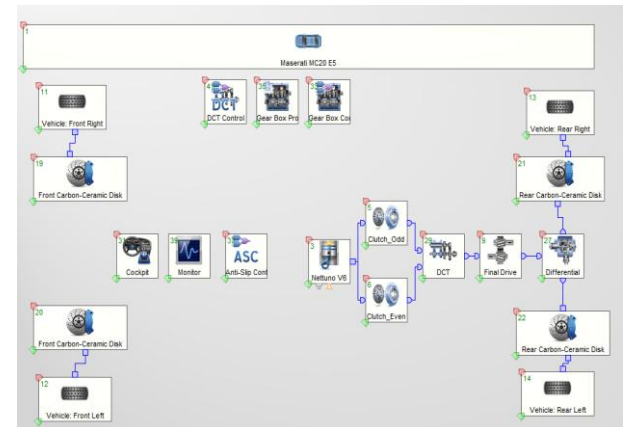
2 pav. „Maserati MC20“, AVL CRUISE modelis Šaltinis: sudaryta autorių
